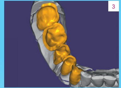
Fig. 3 Sulla struttura in biossido di zirconio realizzata con tecnica CAD/CAM sono state progettate strutture di rivestimento estetico in ceramica ibrida.
